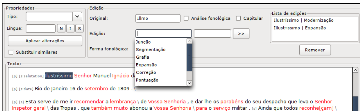
Figura 6. Detalhes da interface de edição de símbolos.
