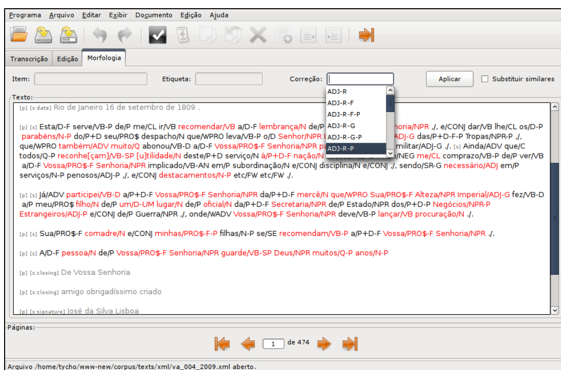
Figura 4. Aba "Morfologia" do E-Dictor.
